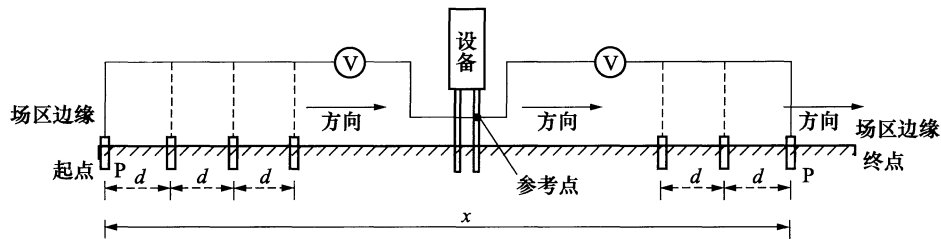
图 5 场区地表电位梯度分布测试示意图
