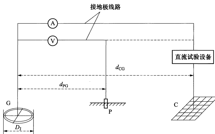
G—直流接地极； D_J —直流接地极外径；P—电位极；C—换流站接地网。
